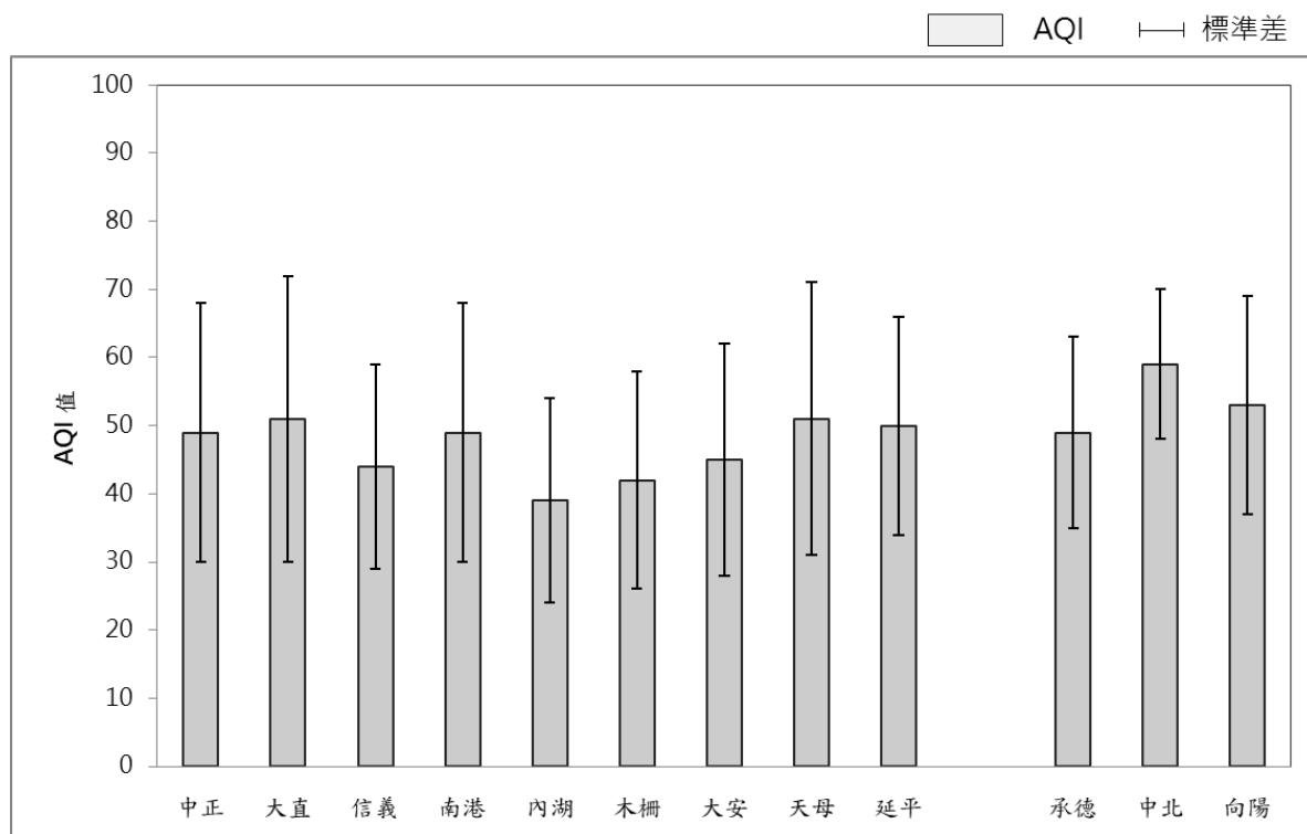
圖 2-1-2 112 年各測站空氣品質指標平均圖
