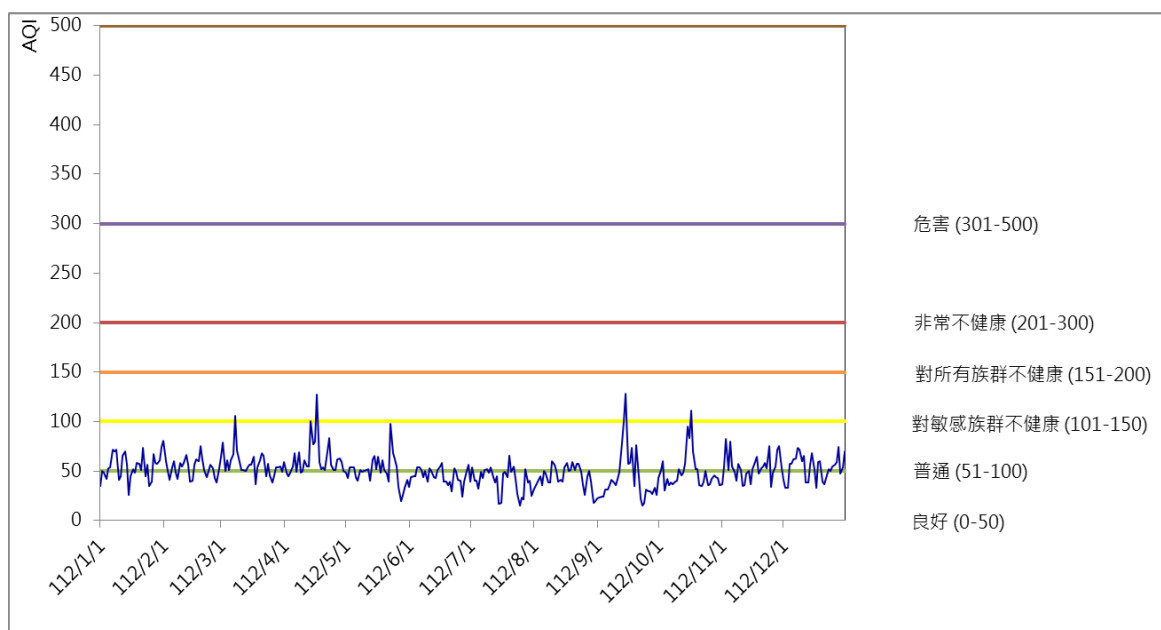
112年延平站每日AQI趨勢圖
