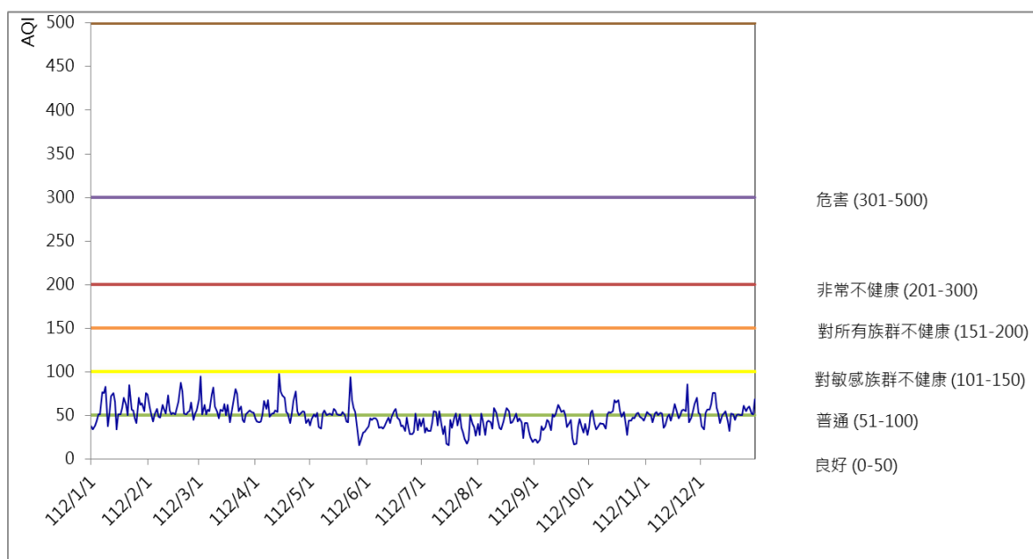
112年承德站每日AQI趨勢圖
