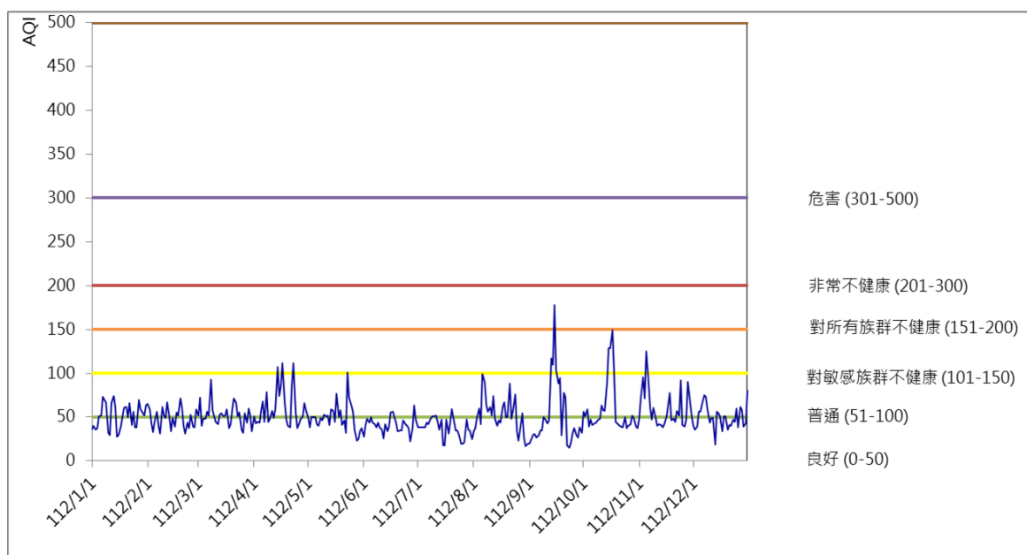
112年信義站每日AQI趨勢圖
