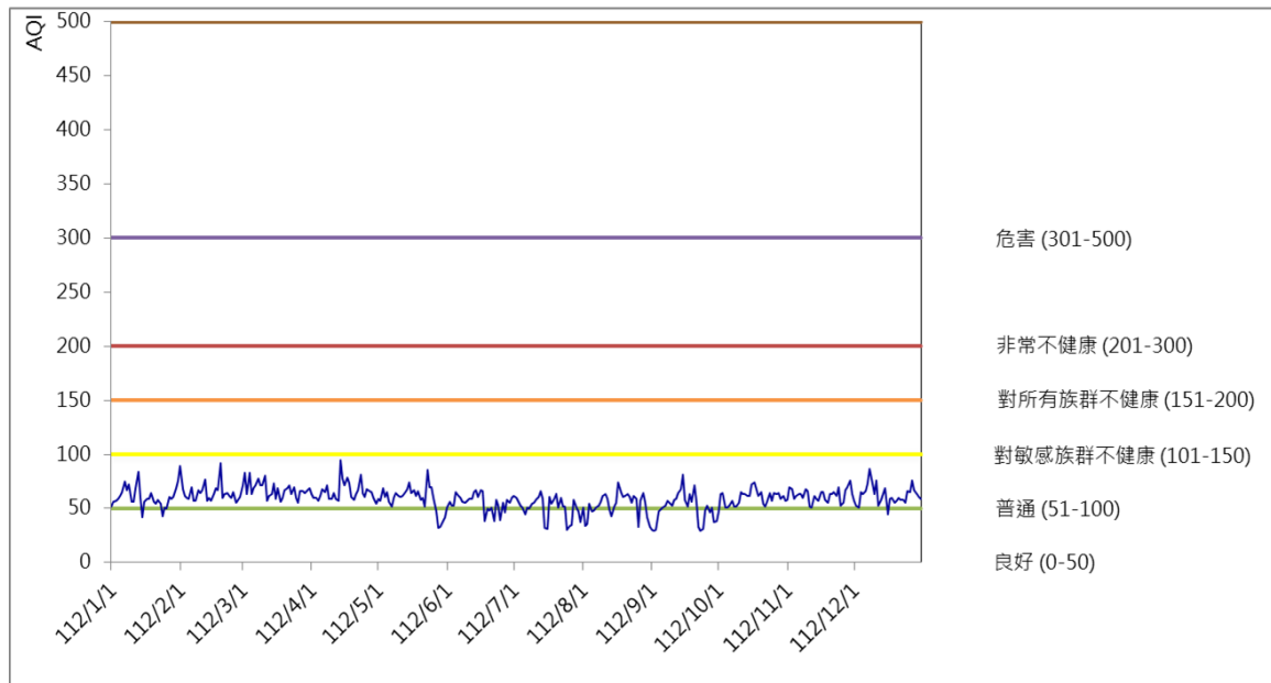
112年中北站每日AQI趨勢圖
