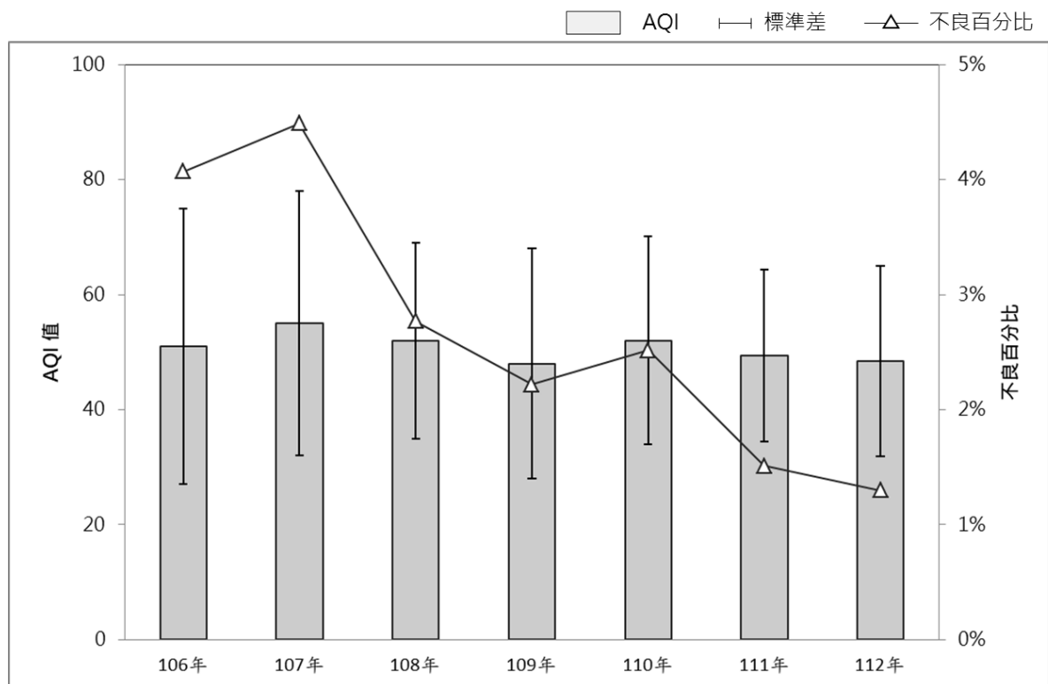
圖 3-1-1 歷年空氣品質指標平均與不良百分比變化圖
