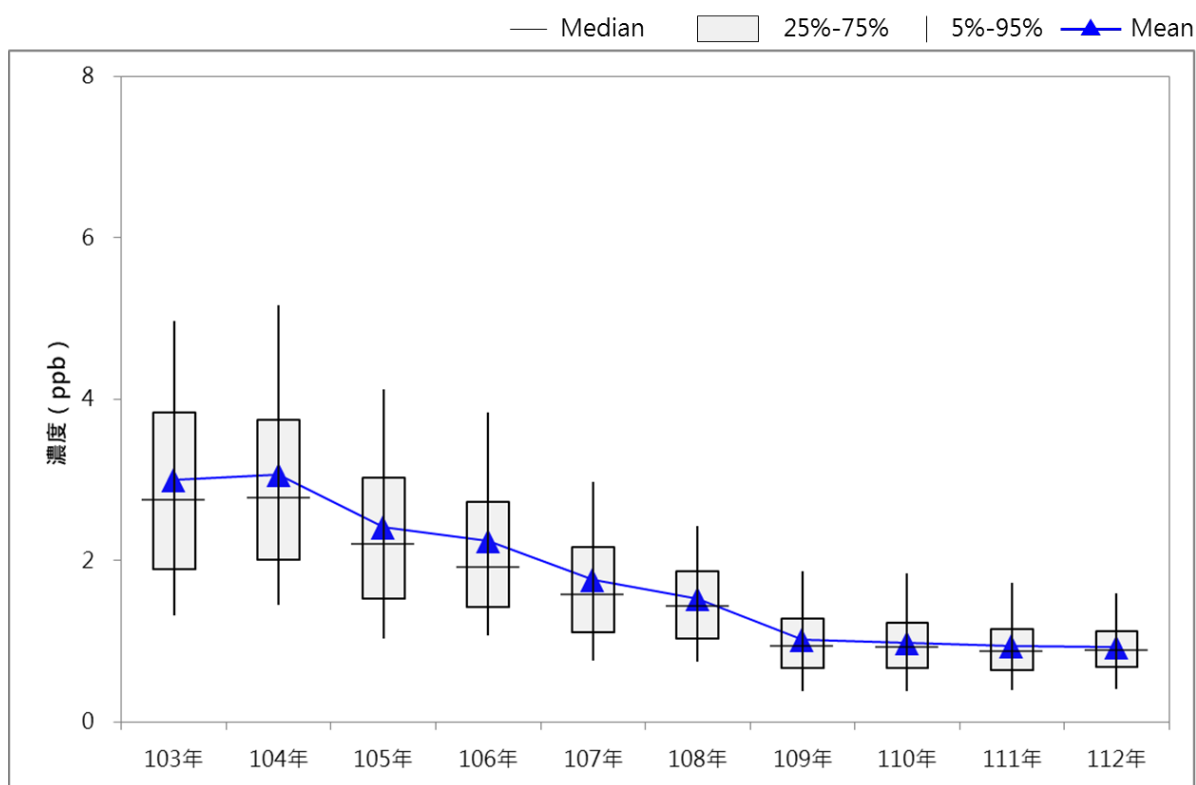
圖 3-2-2 歷年二氧化硫平均濃度趨勢圖
