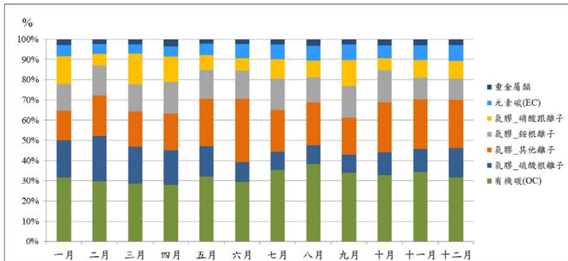
圖 4-2-1 112 年各月份大安站細懸浮微粒成分百分比堆疊圖
