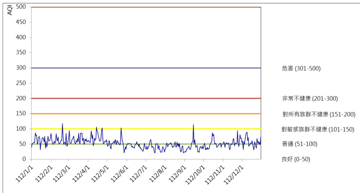
112年向陽站每日AQI趨勢圖
