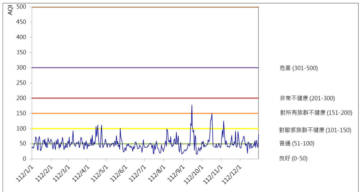
112年大直站每日AQI趨勢圖
