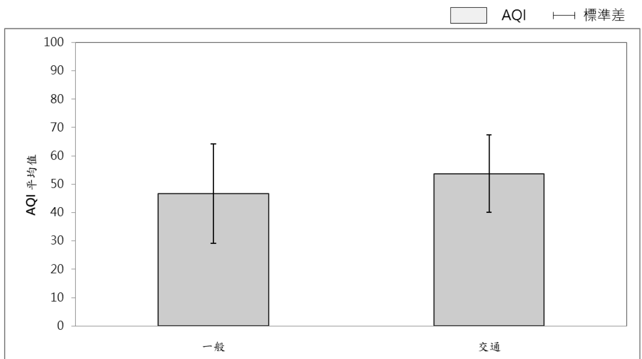
圖 2-1-1 112 年各測站類型空氣品質指標平均圖
