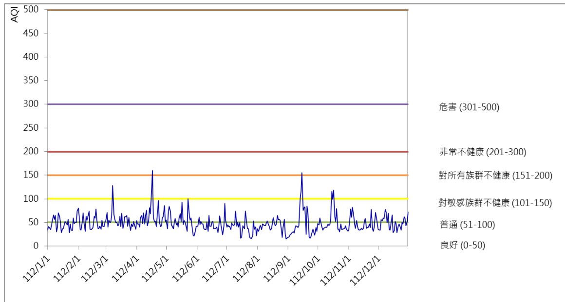
112年中正站每日AQI趨勢圖
