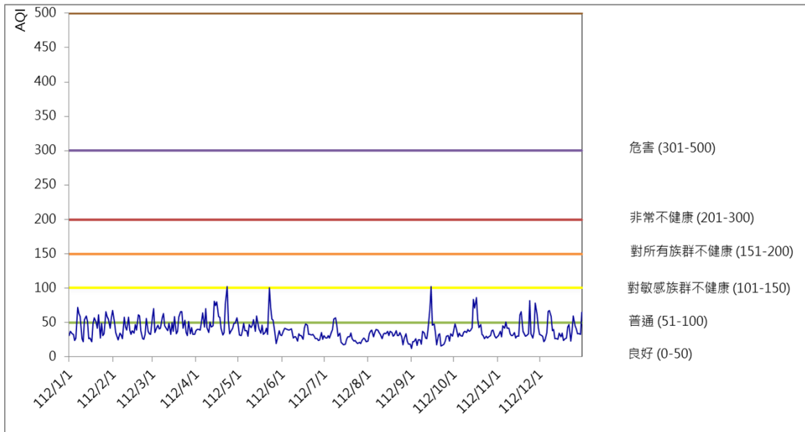
112年內湖站每日AQI趨勢圖
