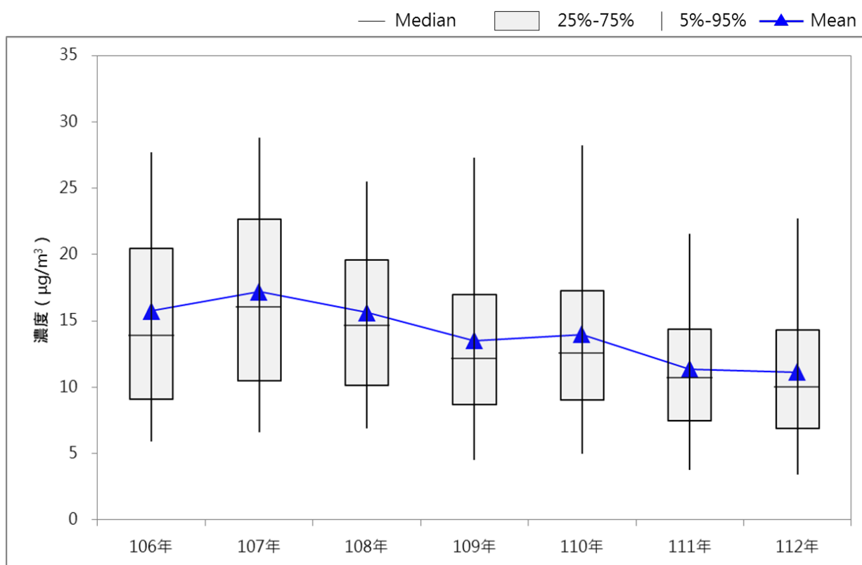
圖 3-2-6 歷年細懸浮微粒（自動監測）平均濃度趨勢圖
