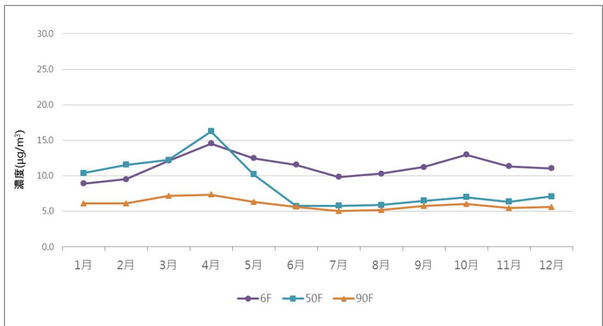
圖 4-1-1 112 年 101 大樓各站細懸浮微粒月平均濃度趨勢圖
