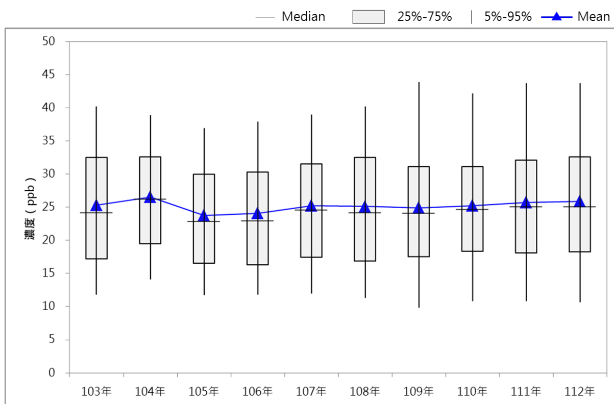
圖 3-2-5 歷年臭氧平均濃度趨勢圖
