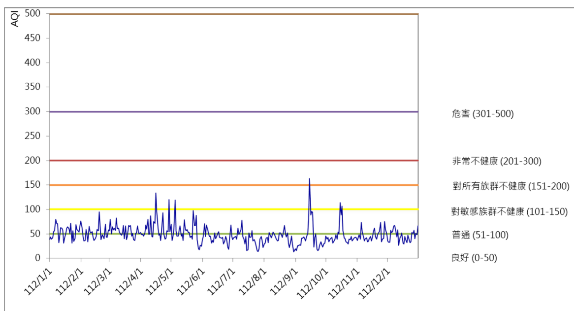
112年南港站每日AQI趨勢圖
