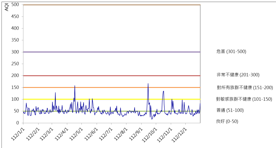
112年天母站每日AQI趨勢圖
