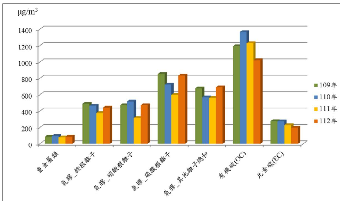
圖 4-2-2 歷年大安站細懸浮微粒各成分項目年累計濃度
