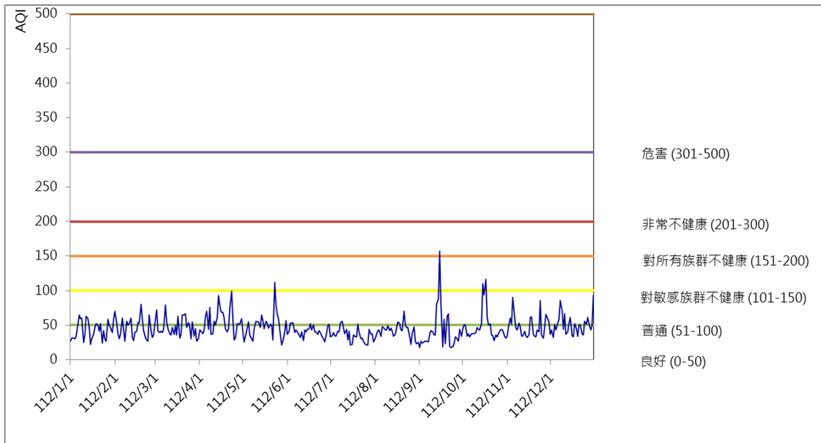
112年大安站每日AQI趨勢圖
