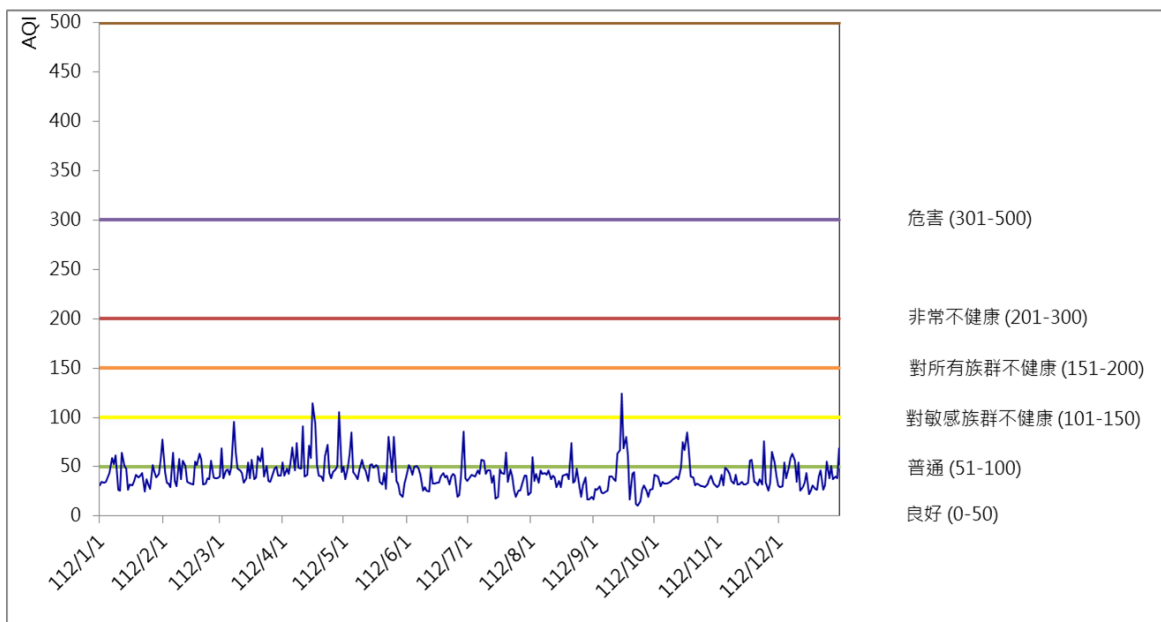
112年木柵站每日AQI趨勢圖
