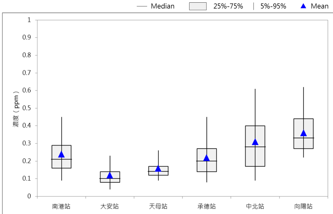
圖 2-2-11 非甲烷總碳氫化合物各測站每日 6-9 時濃度盒鬚圖
