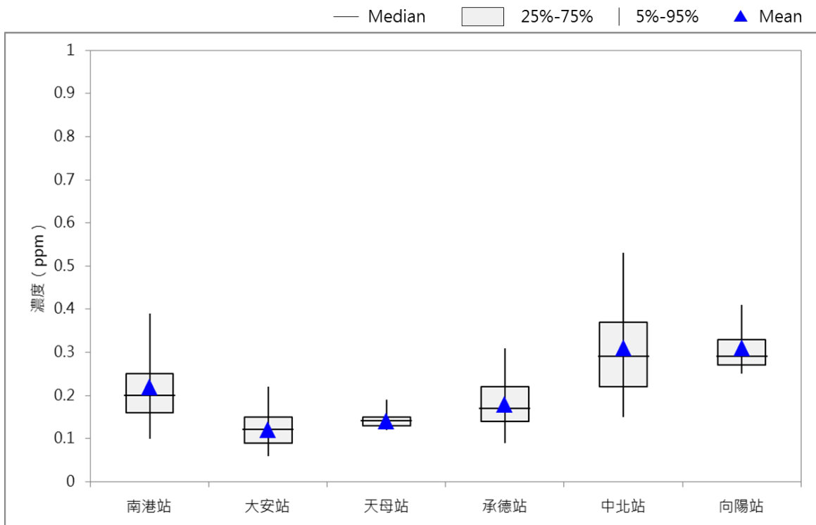
圖 2-2-12 非甲烷總碳氫化合物各測站每日 24 時濃度盒鬚圖
