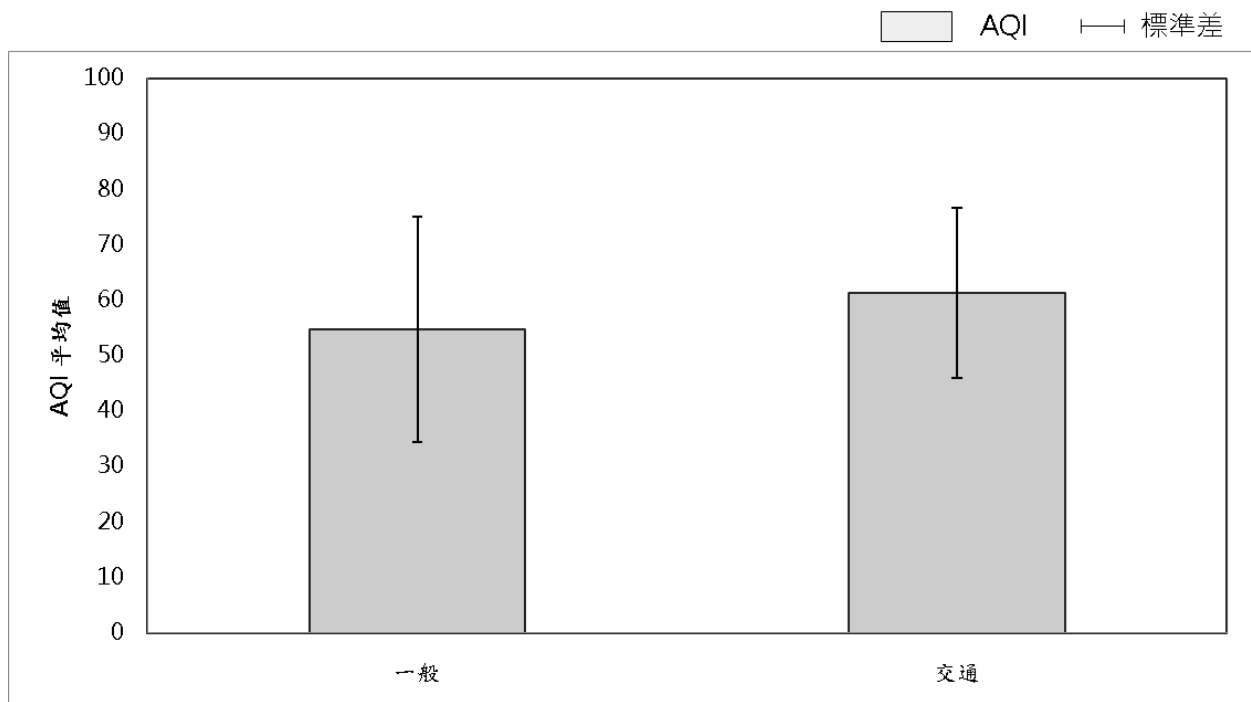
圖 2-1-1 114 年各測站類型空氣品質指標平均圖
