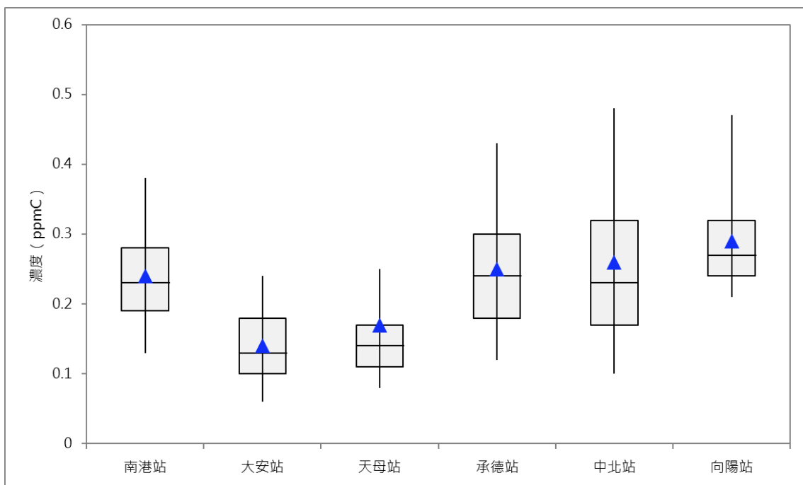
圖 2-2-11 非甲烷碳氫化合物各測站每日 6-9 時濃度盒鬚圖
