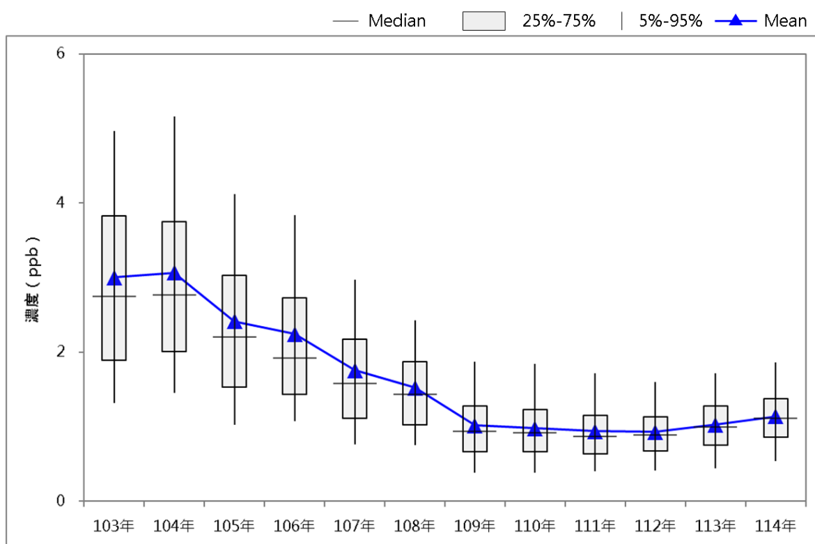
圖 3-2-2 歷年二氧化硫平均濃度趨勢圖
