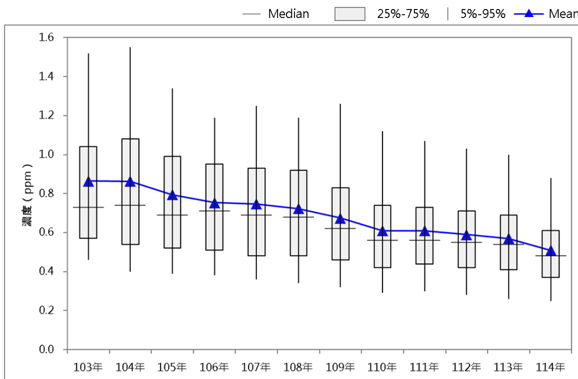
圖 3-2-4 歷年一氧化碳平均濃度趨勢圖
