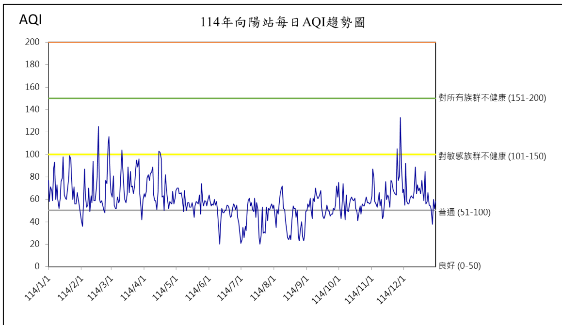
圖 2-1-3 (A) 中正 (B) 大直 (C) 信義 (D) 南港 (E) 內湖 (F) 木柵 (G) 大安 (H) 天母 (I) 延平 (J) 承德 (K) 中北 (L) 向陽測站空氣品質指標趨勢圖
