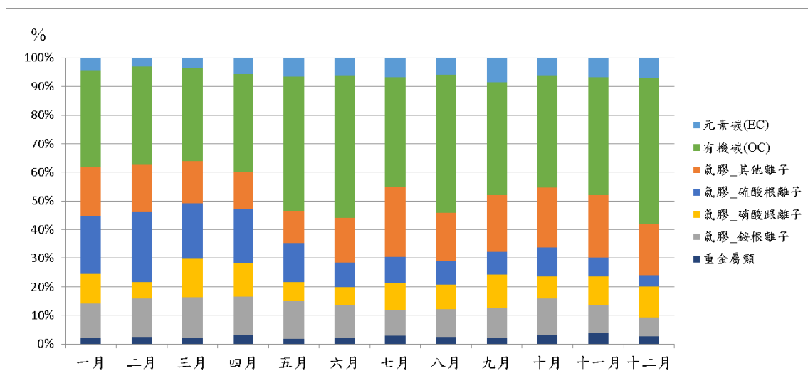
圖 4-2-1 114 年各月份大安站細懸浮微粒成分百分比堆疊圖
