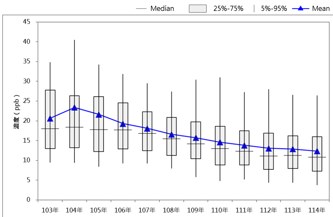
圖 3-2-3 歷年二氧化氮平均濃度趨勢圖
