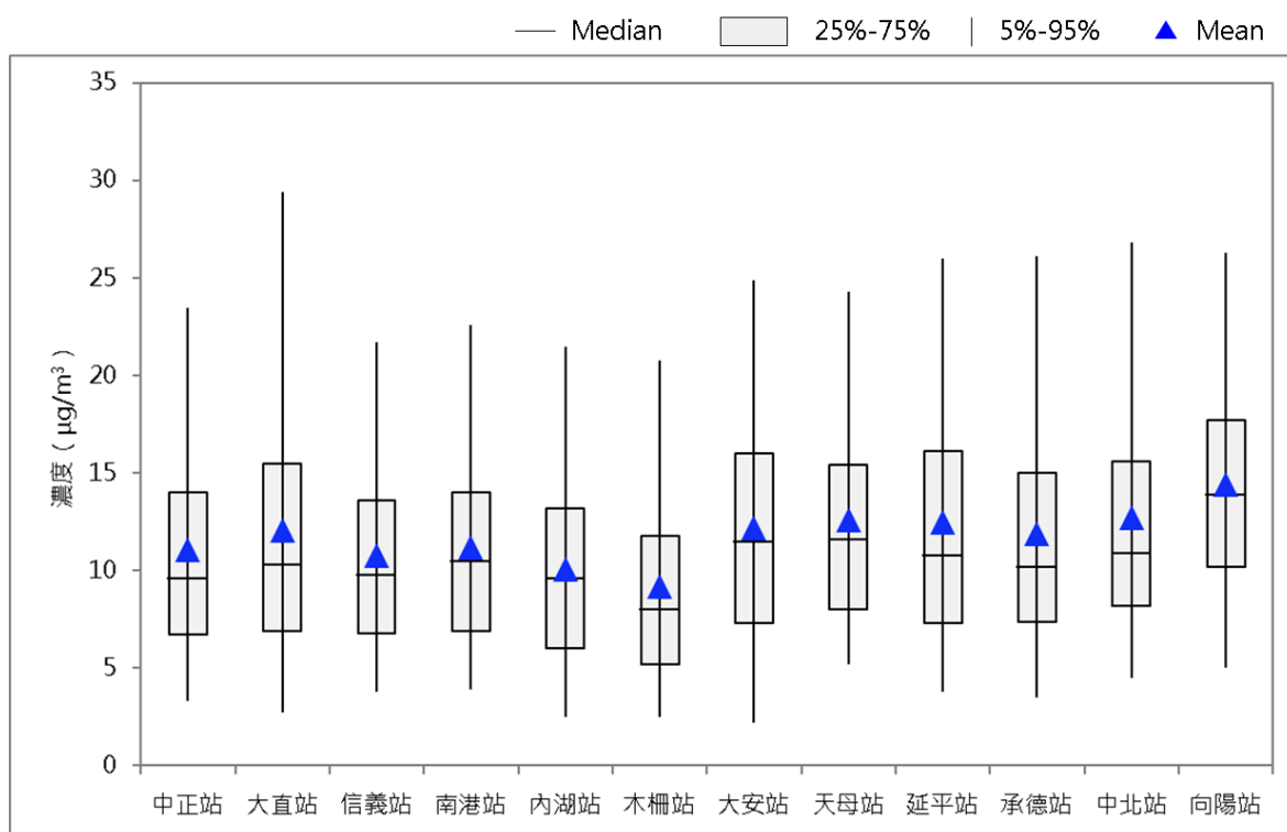
圖 2-4-1 細懸浮微粒自動監測 (A) 測站類型 (B) 各測站濃度盒鬚圖
