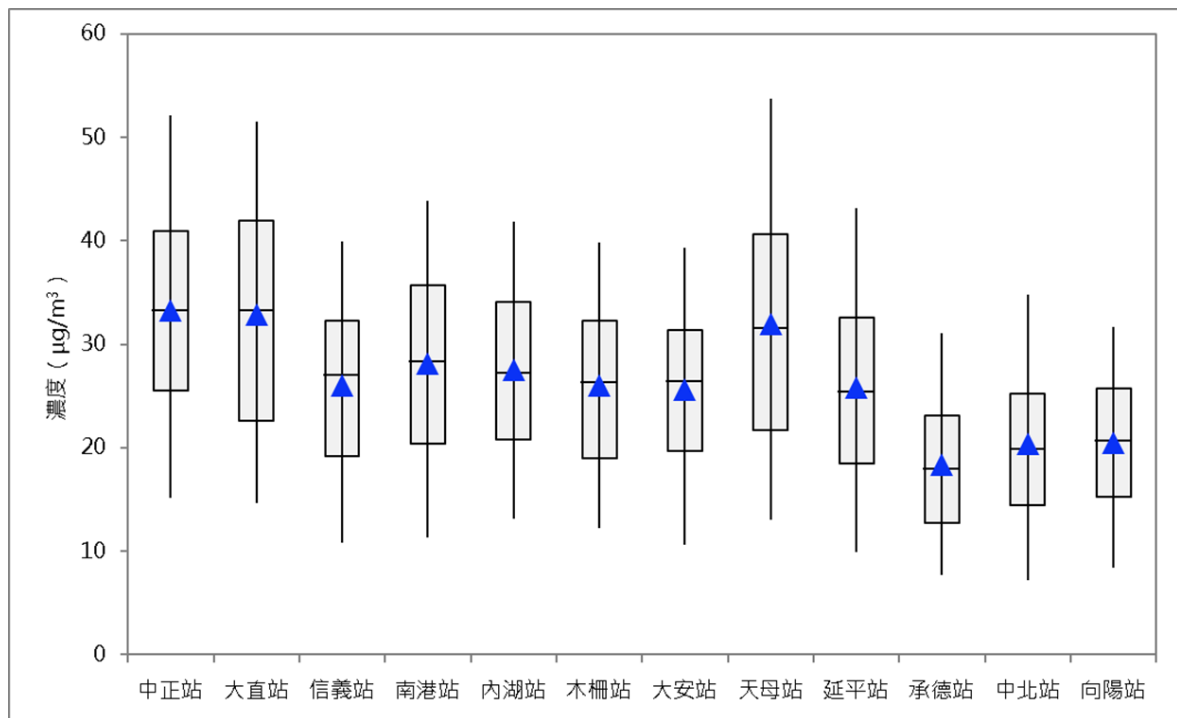
圖 2-2-5 臭氧 (A) 測站類型 (B) 各測站平均濃度盒鬚圖
