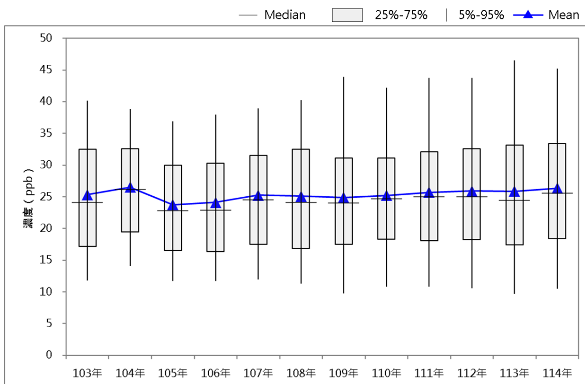
圖 3-2-5 歷年臭氧平均濃度趨勢圖
