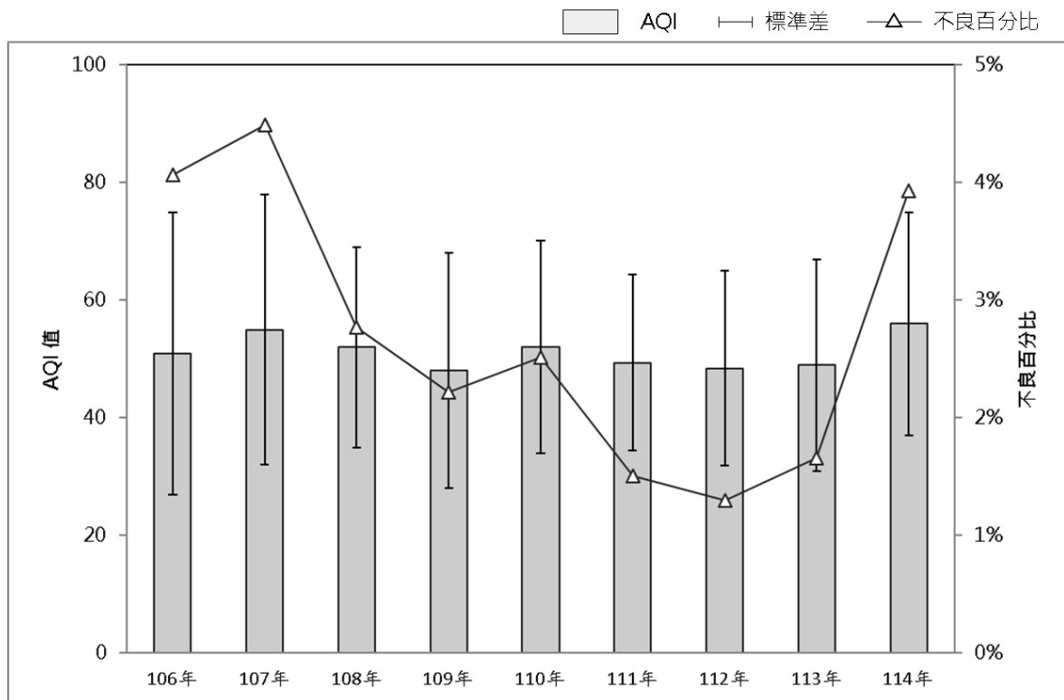
圖 3-1-1 歷年空氣品質指標平均與不良百分比變化圖
