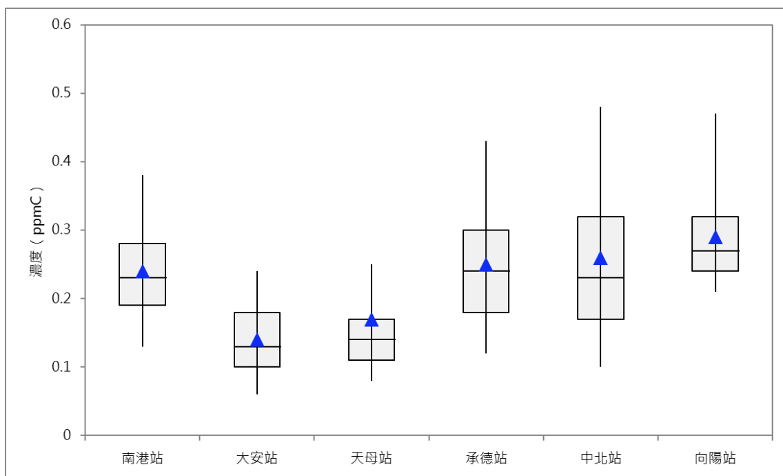
圖 2-2-12 非甲烷碳氫化合物各測站每日 24 時濃度盒鬚圖
