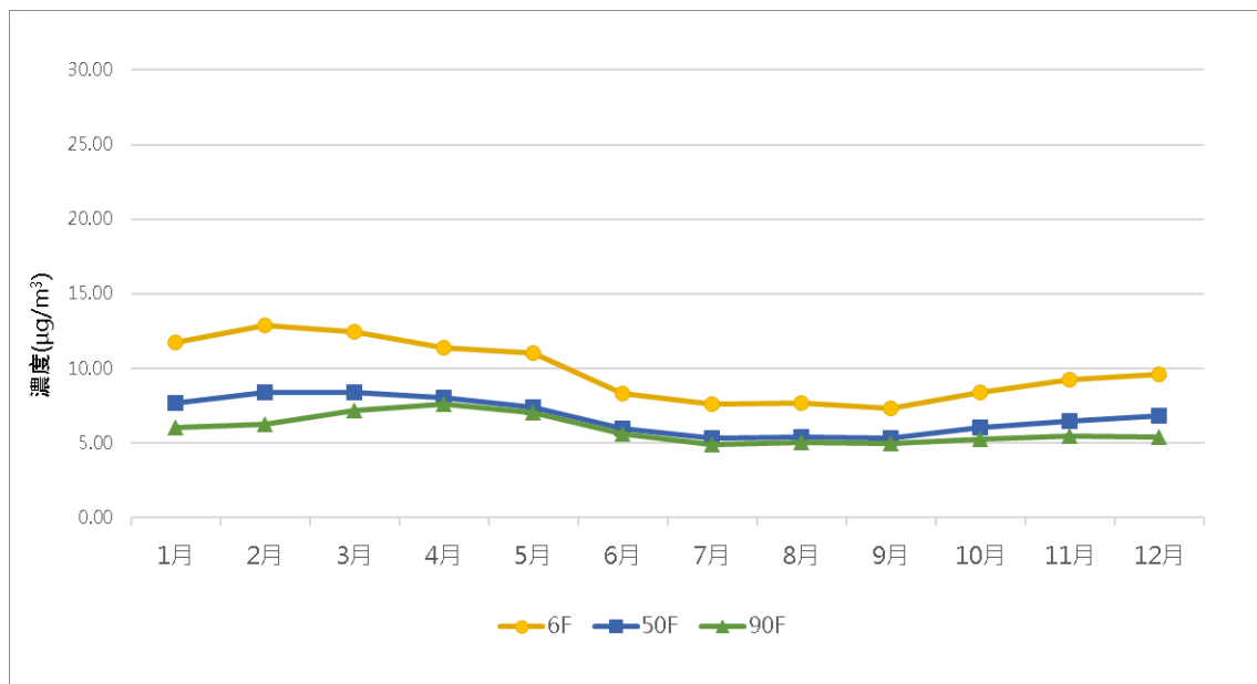
圖 4-1-1 114 年 101 大樓各站細懸浮微粒月平均濃度趨勢圖
