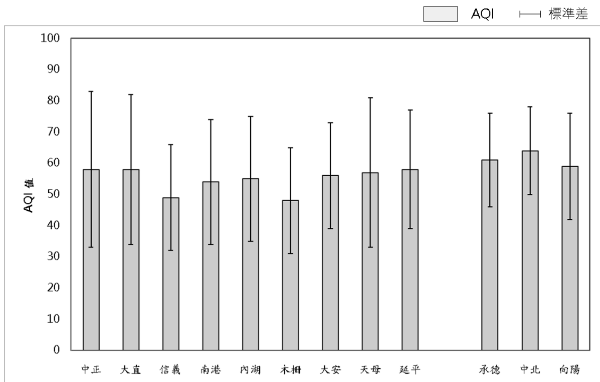
圖 2-1-2 114 年各測站空氣品質指標平均圖
