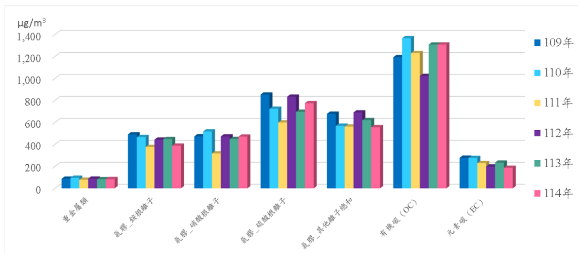
圖 4-2-2 歷年大安站細懸浮微粒各成分項目年累計濃度
